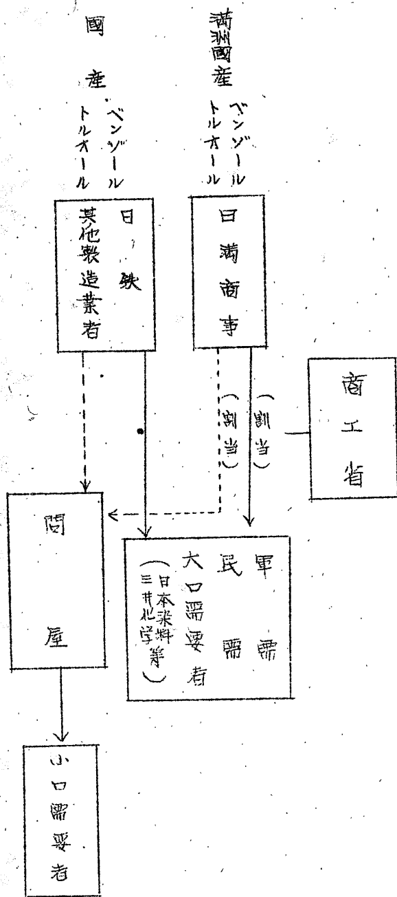
ベンゾール及トルオールノ配給系統図
