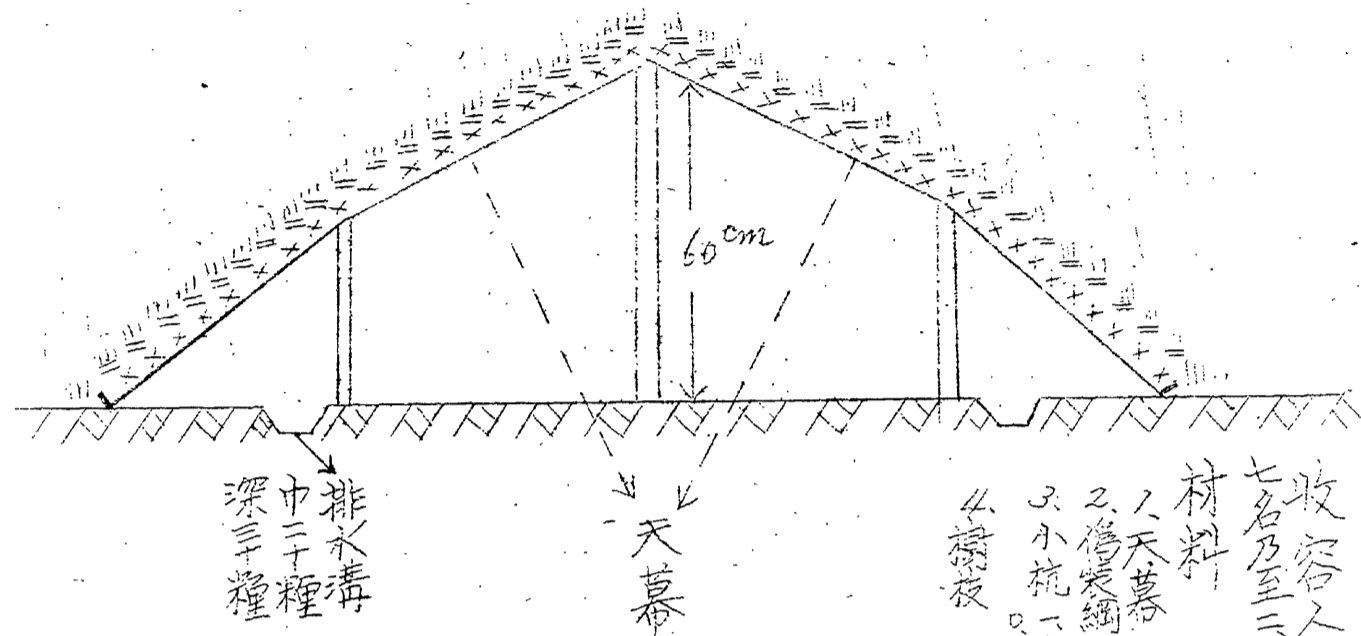
断面圖
