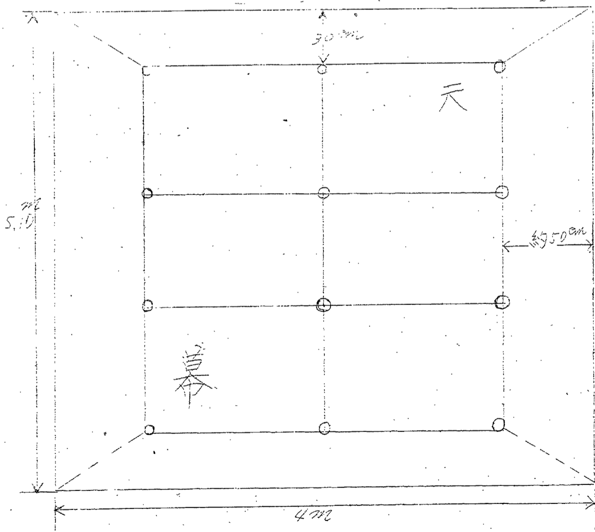
平面圖
