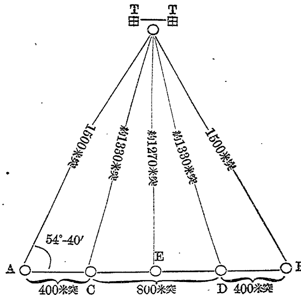
航路圖 甲 (十二斤砲以上ニ用ユル者)
