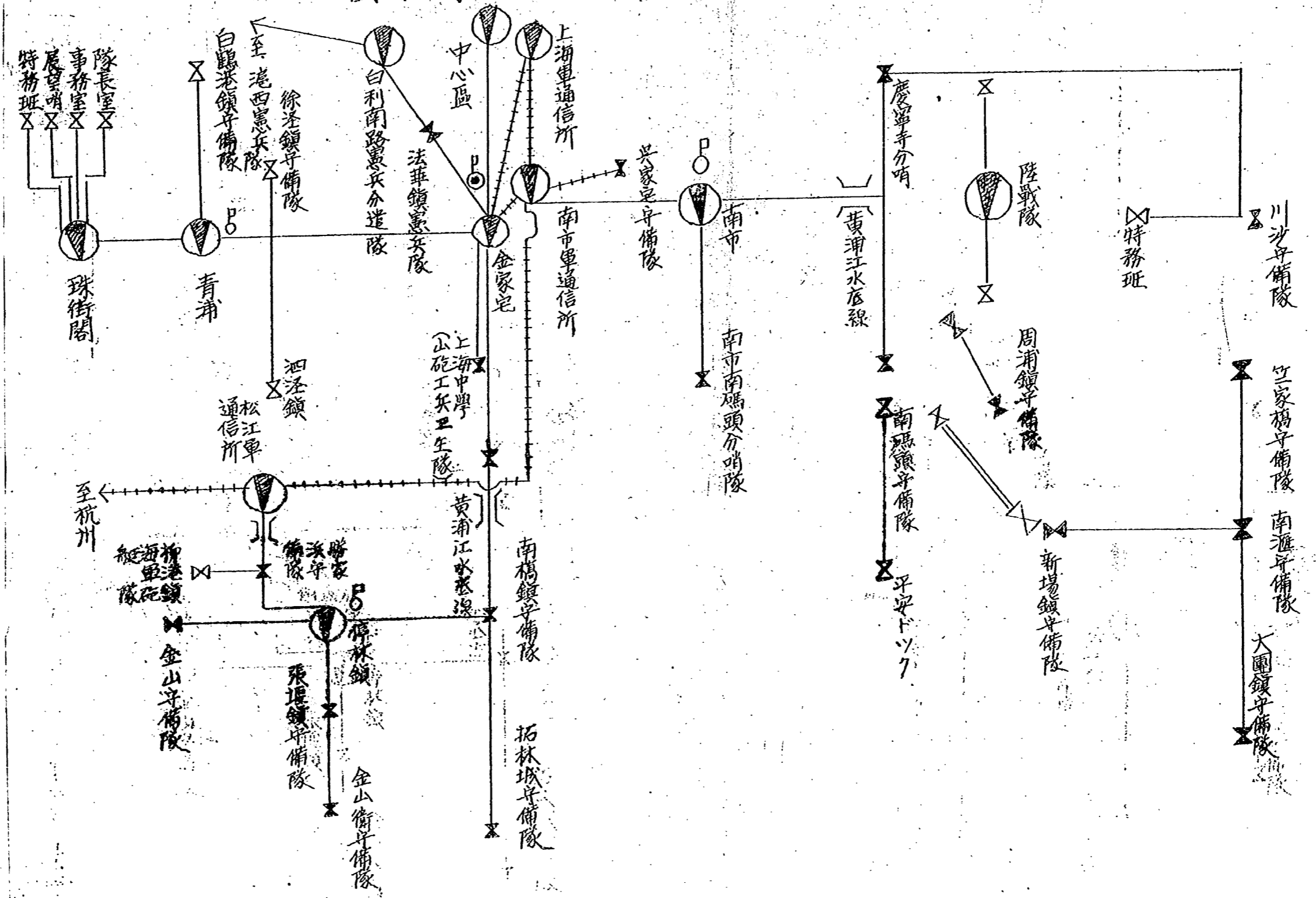
上海南地區警備隊有線通信網要圖
