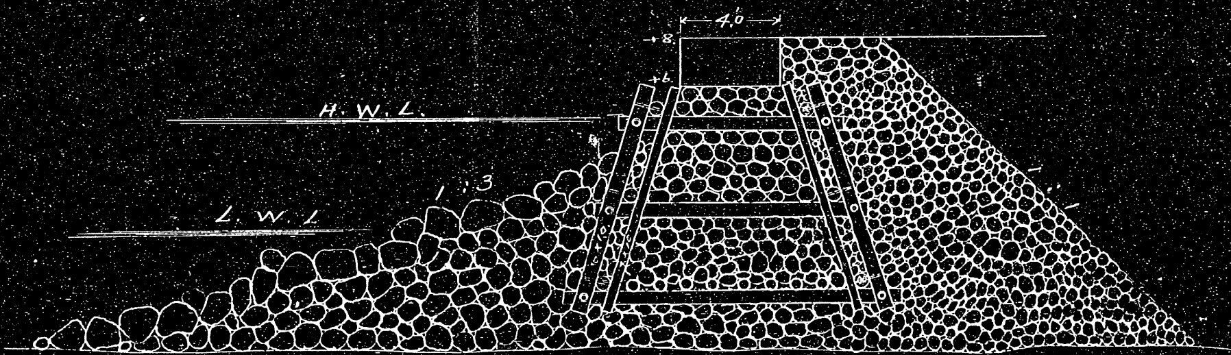
埋立護岸(乙)
