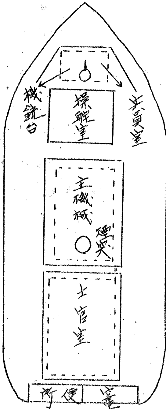
艦載水雷艇略圖
