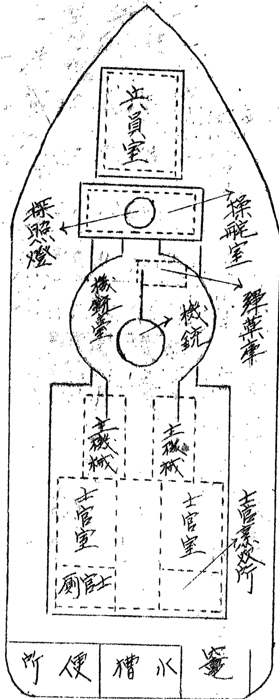
中形砲艇略圖
