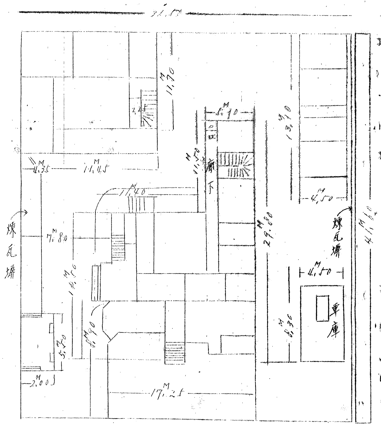
二階平面図縮尺 \frac{1}{200}
