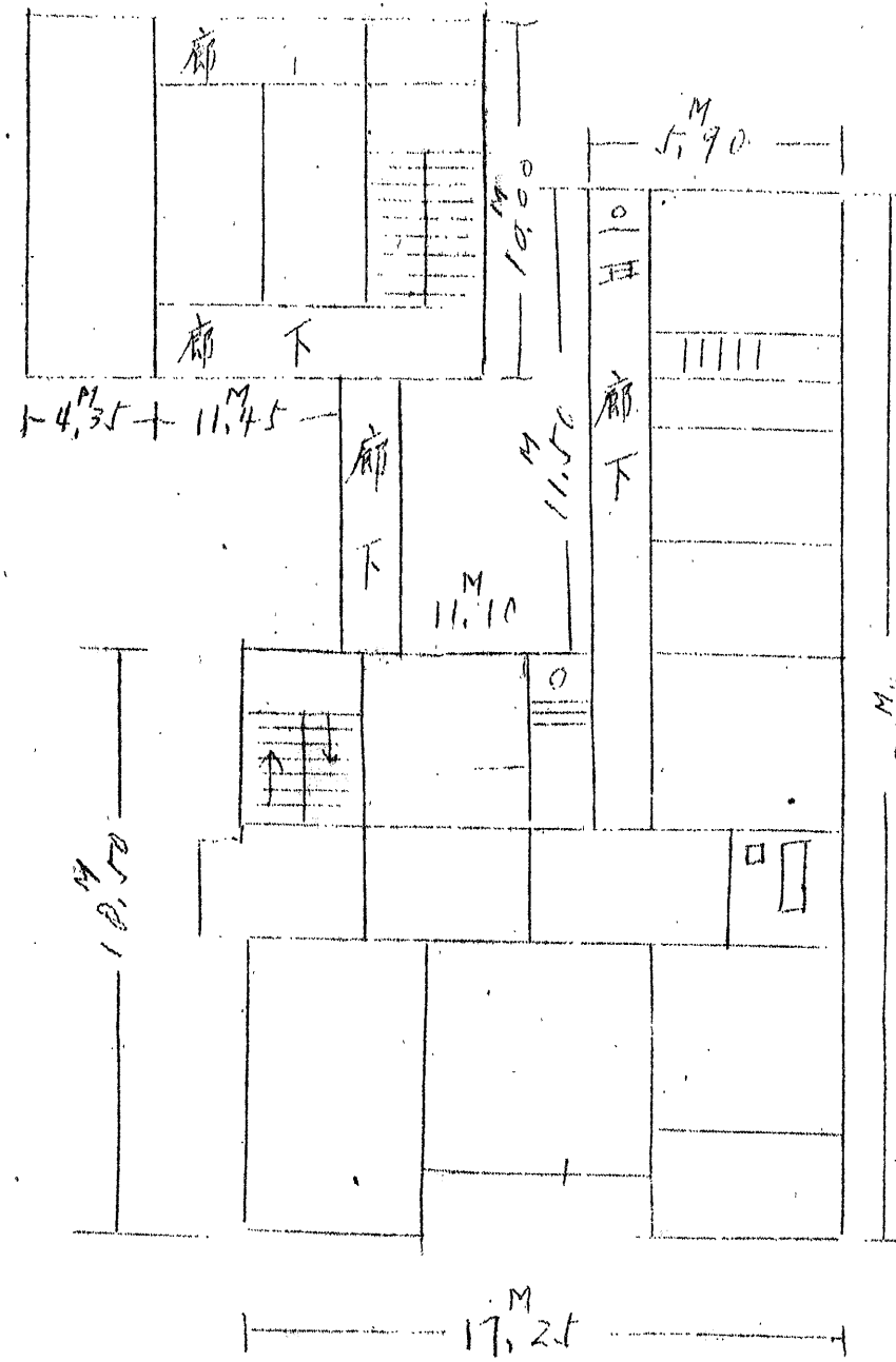
二階平面図縮尺 \frac{1}{200}
