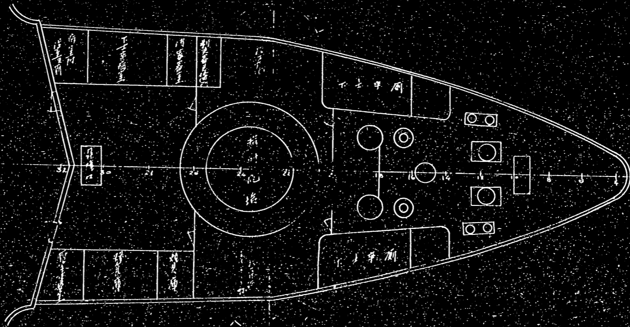
上甲板平面
