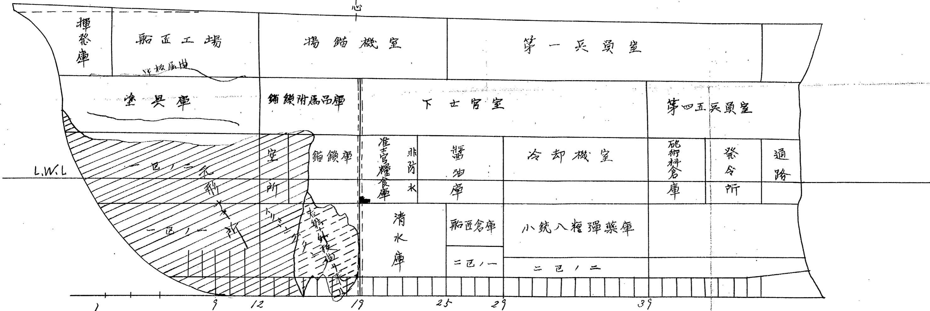
船艙甲板平面
