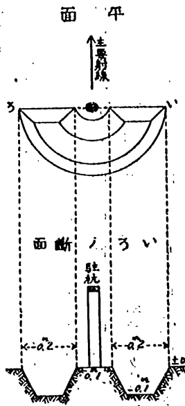
單砲效線 砲床準備及掘砲
