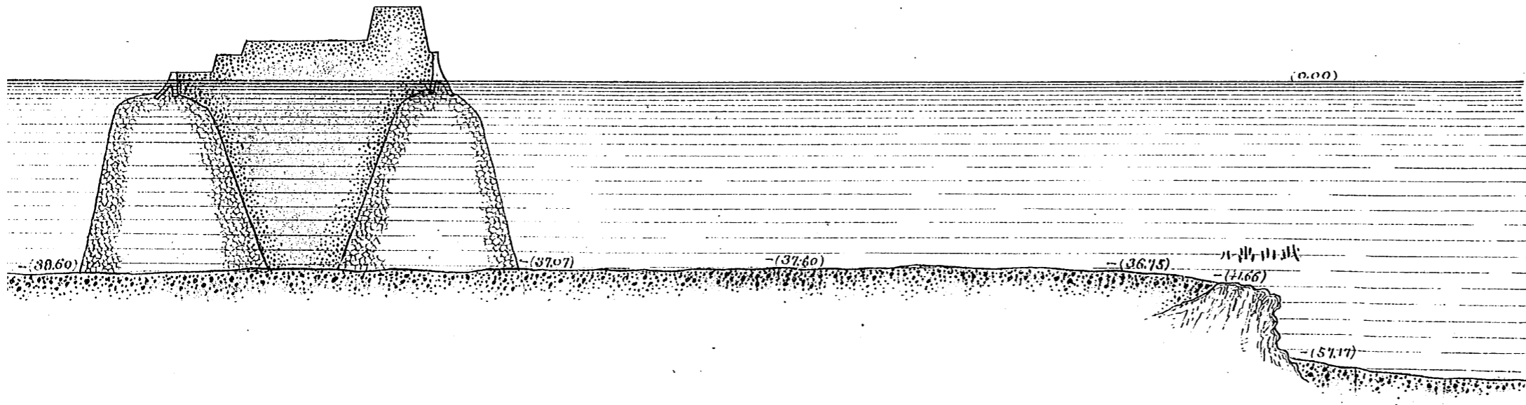
AB 之 断 面
