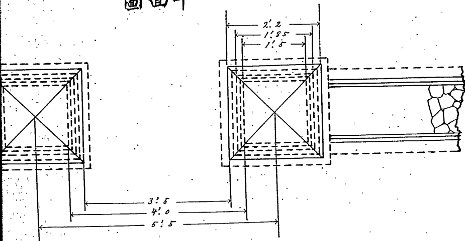
平面圖
