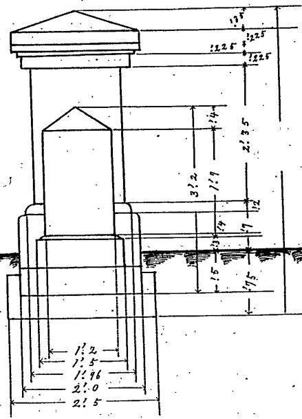
橫斷面圖
