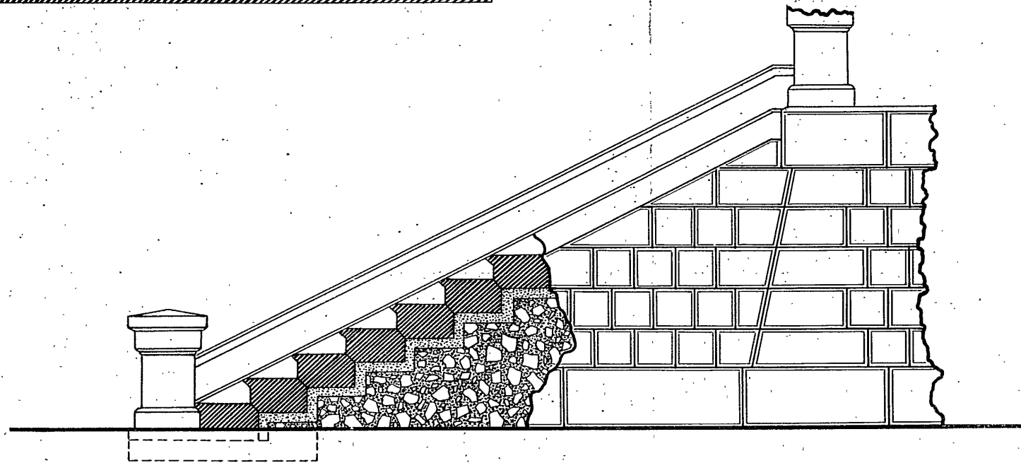
圖面側段階
