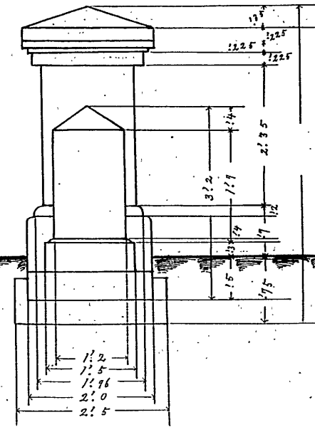
橫斷面圖
