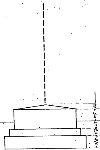
圖面正
