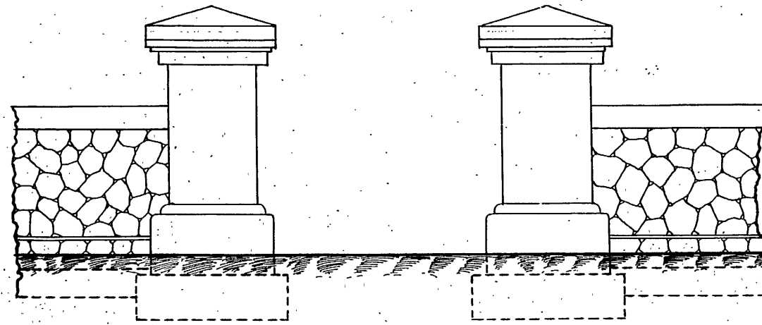
正面圖
