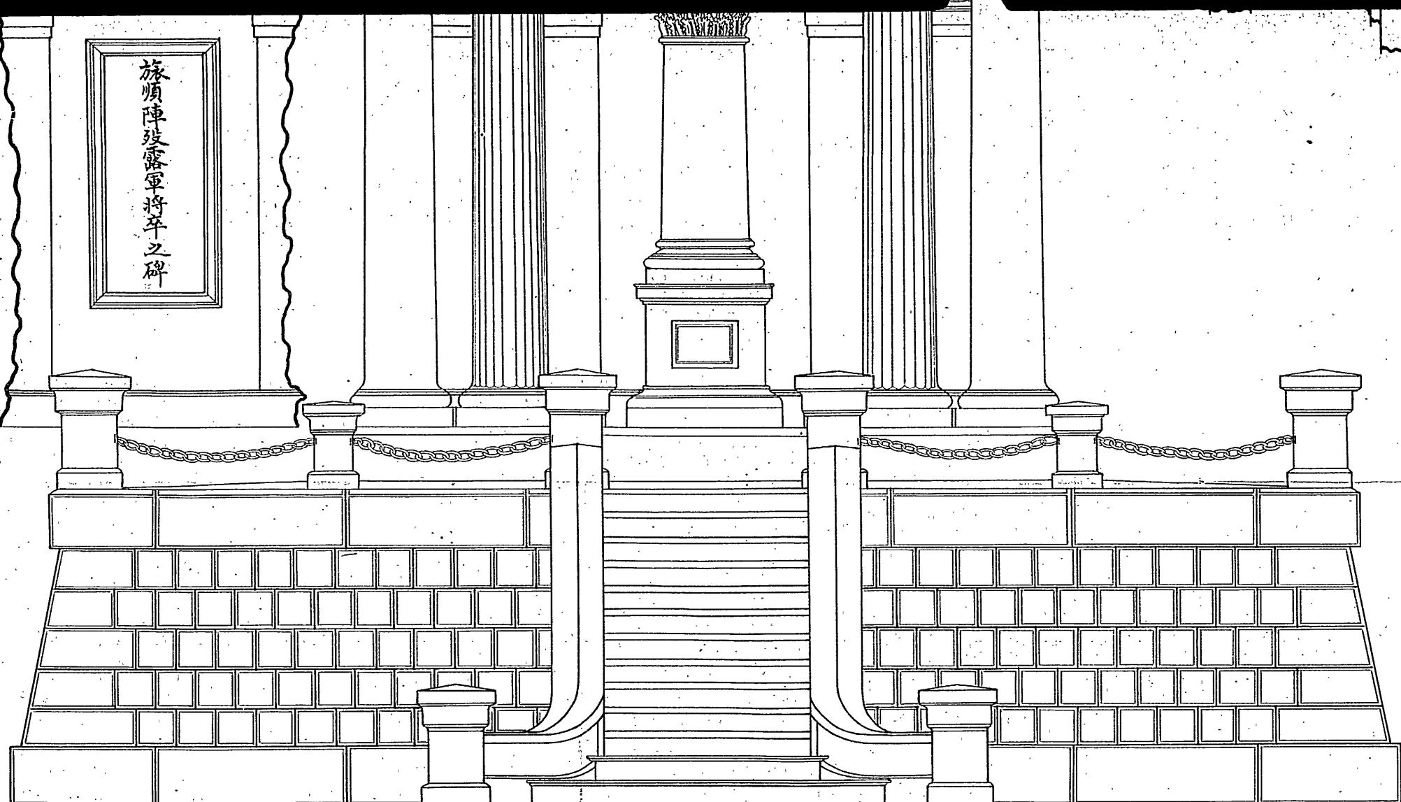
圖面正
