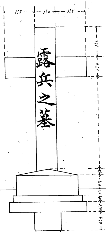
正面圖
