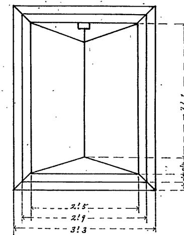
圖面平
