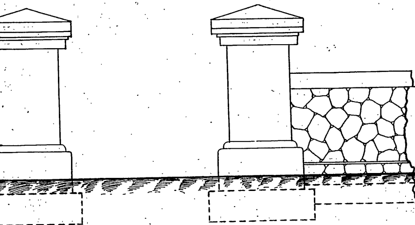
正面圖
